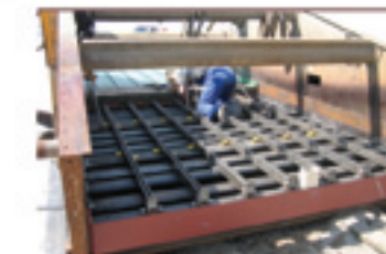
Austausch Geweberahmen im Kieswerk
